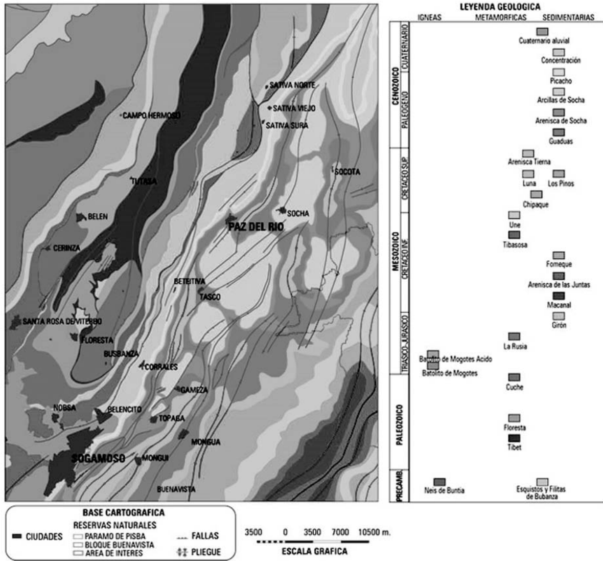
FIGURA 2. Mapa geológico de la zona de estudio. Bloque Soapaga. Cordillera Oriental. Tomado de www.rondacolombia2008/img/secciones/cuenca/cordillera/marco_1.jpg . Elaborado por Andreas Kammer.
