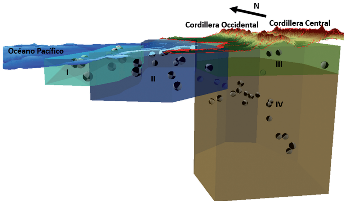
FIGURA 6. Esquema tridimensional de los mecanismos focales de los terremotos para los cuatro ambientes tectónicos determinados.
