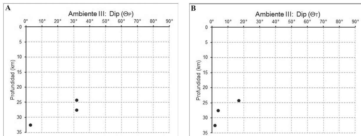
FIGURA 9. Representación de los ángulos de inmersión ( Plunge ) de los ejes de esfuerzos, A. Compresivo ( P ) y B. Tensión ( T ) en el Ambiente Sismotectónico III, zona continental superficial.
