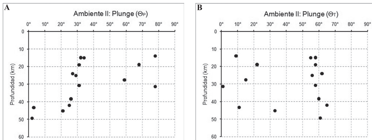
FIGURA 8. Representación de los ángulos de inmersión (Plunge) de los ejes de esfuerzos, A. Compresivo ( P ) y B. Tensión ( T ) en el Ambiente Sismotectónico II, zona de flexión e interacción interplacas.
