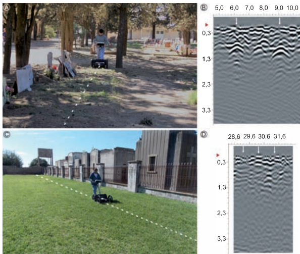
FIGURA 8. A. Vista inhumaciones sector oeste cementerio. B. Radargrama con reflexiones hiperbólicas de fértros, las flechas indican la ubicación de los mismos. C. Vista patio interior cementerio. D. Radargrama donde se indican con flechas las fosas vacías.
