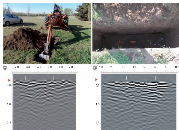
FIGURA 7. A. Vista excavación fosa simulada. B. Foto de una vista superior de la fosa. C. Radargrama 14-Set-2016. D. Radargrama 14-Feb-2017. En ambos las flechas indican los límites interpretados de la fosa.
