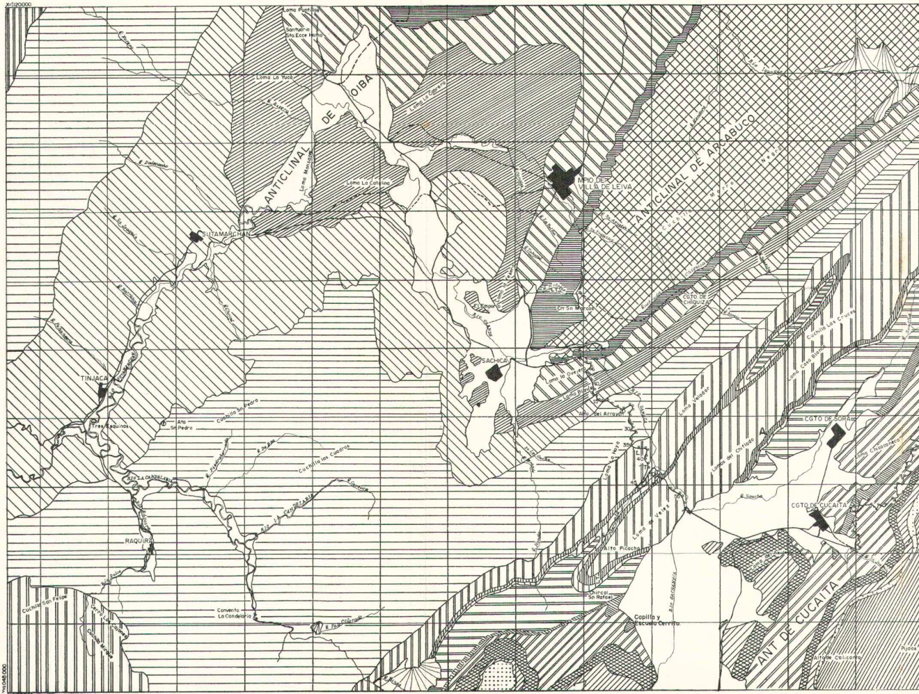
REPUBLICA DE COLOMBIA MINISTERIO DE MINAS Y PETROLEOS - SERVICIO GEOLOGICO NACIONAL MAPA GEOLOGICO DE LA REGION DE VILLA DE LEIVA Y ZONAS PROXIMAS Fernando Etayo Serna 1965
