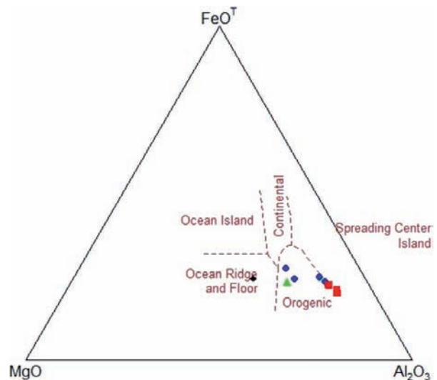
FIGURA 15. Diagrama de Al_2O_3 -MgO- FeO^T , proporciones moleculares de las muestras, de Pearce et al. (1984). Azul=gabros, rojo=dacitas, verde=andesitas.
