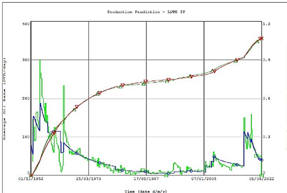
Figura 9. Ajuste histórico de producción de petróleo y su acumulado.
