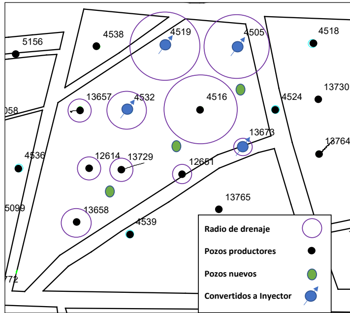
Figura 16. Mapa de ubicación de pozos, radios de drenaje y conversión de pozos productores a inyector.
