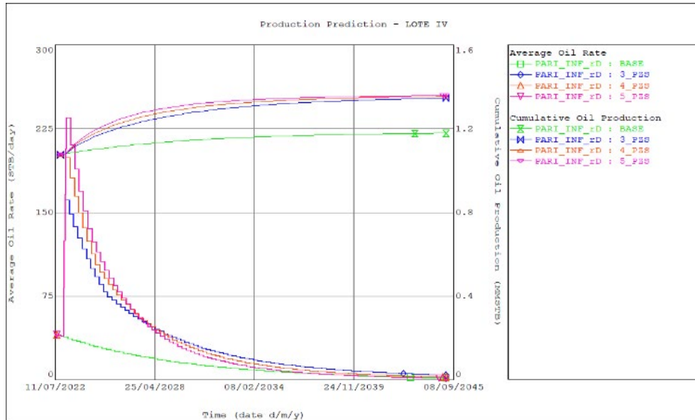
Figura 13. Predicciones Base e incrementales de perforación de 3, 4 y 5 pozos.
