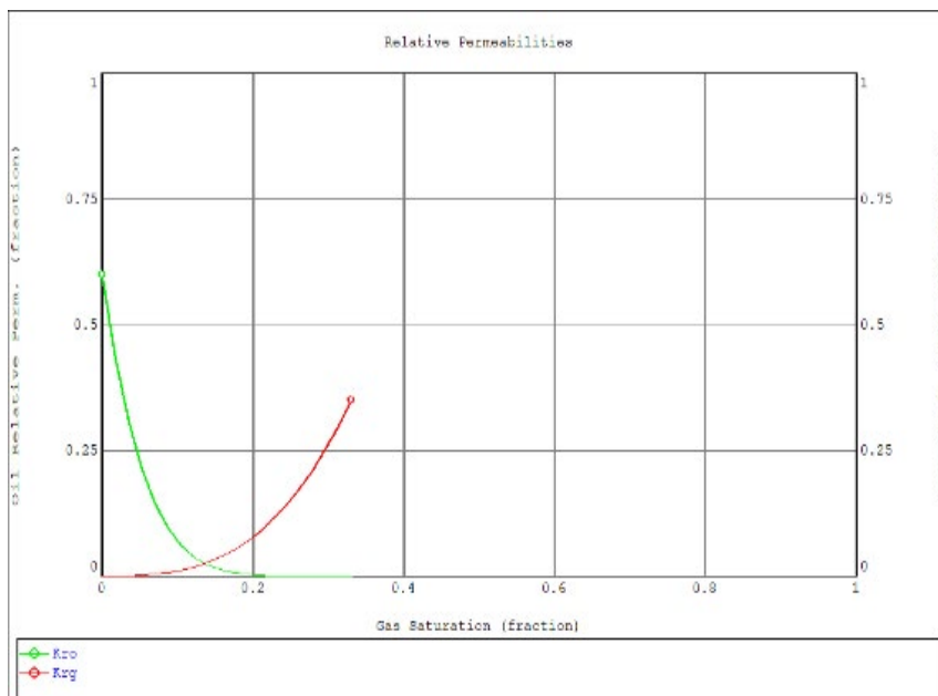
Figura 8. Curvas de Corey “Kro vs Krw” y “Kro vs Krg” usadas en el modelo.
