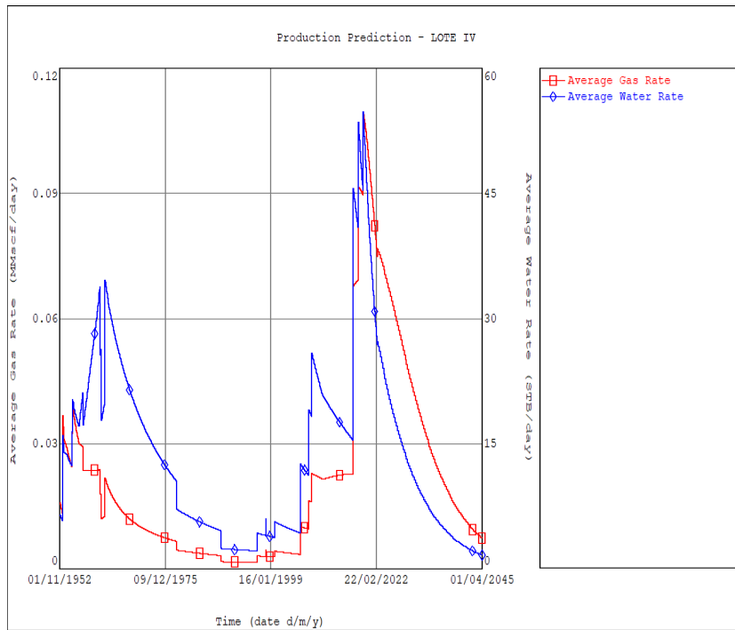
Figura 11b. Caso Base: Producción de agua y gas.
