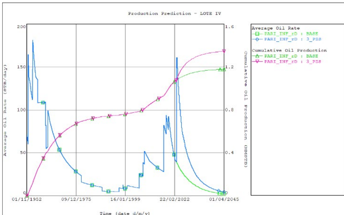
Figura 12. Predicciones de curva Base + perforación de 3 pozos.
