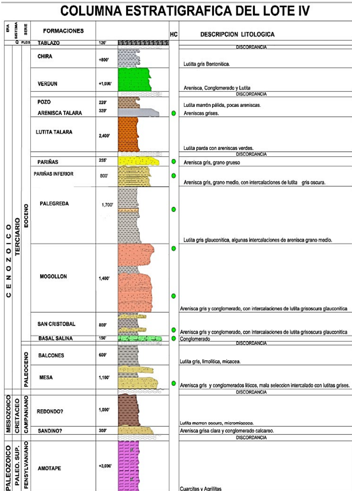
Figura 2. Columna estratigráfica compuesta del Lote IV - Zona "A".
