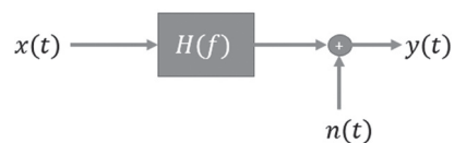
Figura 1. Representación de un sistema lti para un canal plc.
