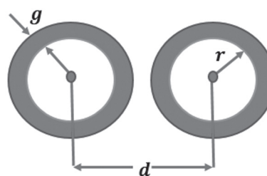
Figura 12. Sección transversal de una línea bifilar asociada al cableado eléctrico en ambientes residenciales
