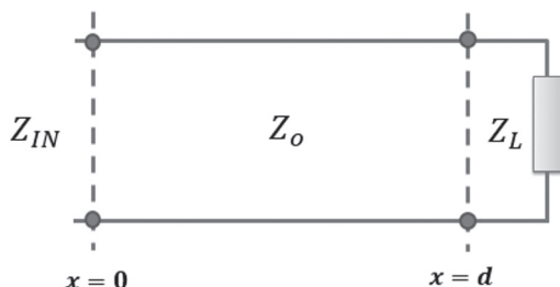
Figura 11. Traslación de impedancia en una sección al interior de una línea de transmisión
