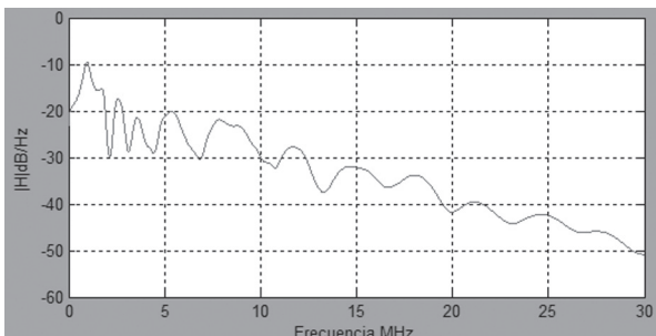
Figura 17. Respuesta de canal plc en condiciones deficientes
