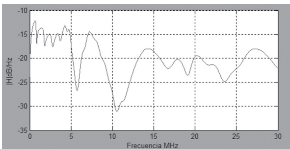
Figura 16. Respuesta de un canal plc en condiciones típicas
