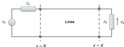
Figura 7. Línea de transmisión terminada
