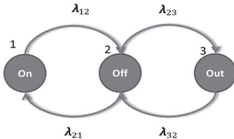
Figura 4. Modelo markoviano tri-estado para dispositivos eléctricos.
