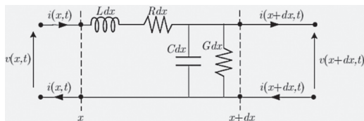
Figura 8. Representación diferencial de una línea de transmisión
