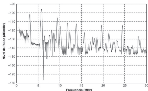
Figura 13. Nivel de ruido en un canal plc
