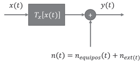
Figura 5. Modelo general del comportamiento del canal
