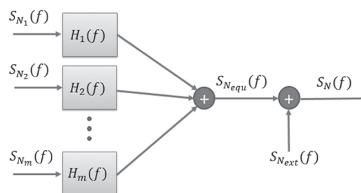
Figura 14. Esquema general del ruido en el receptor.
