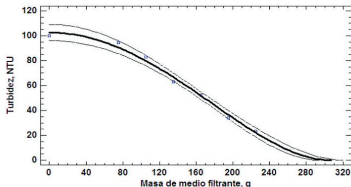
Figura 3. Gráfico de la relación entre la Turbidez y las cantidades de cáscara de coco utilizadas en los tratamientos
