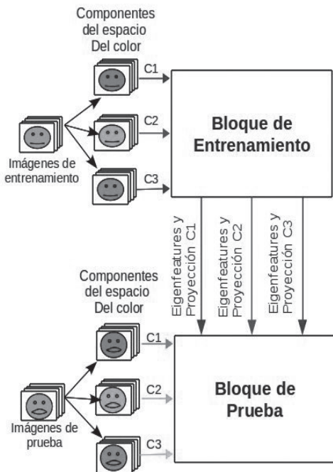
Figura 5. Estructura del sistema de reconocimiento facial.
