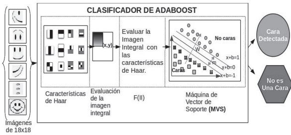
Figura 4. Estructura del sistema de clasificación débil para detectar rostros.
