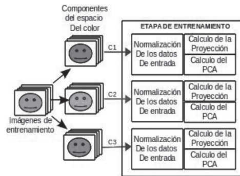
Figura 6. Bloque de Entrenamiento.
