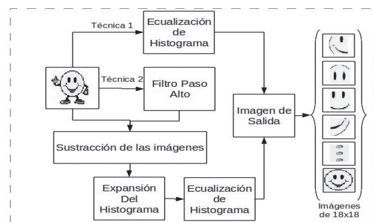
Figura 2. Modelo de las Técnicas de Pre-Procesamiento Digital de Imágenes.
