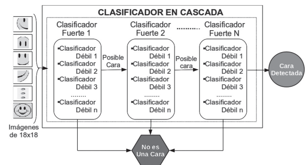
Figura 3. Estructura del sistema clasificador en cascada.
