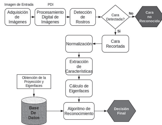
Figura 1. Estructura del Sistema de Detección y Reconocimiento de Rostros.
