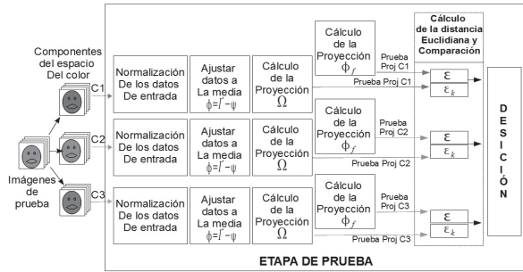
Figura 8. Etapa de Prueba aplicando la Distancia de Euclidiana.
