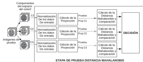
Figura 7. Etapa de Prueba aplicando la Distancia de Mahalanobis.
