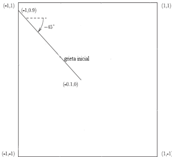
Figura 3. Grieta inicial del caso de referencia de Dufлот, [10]. Fuente. Elaboración modificada de [10].
