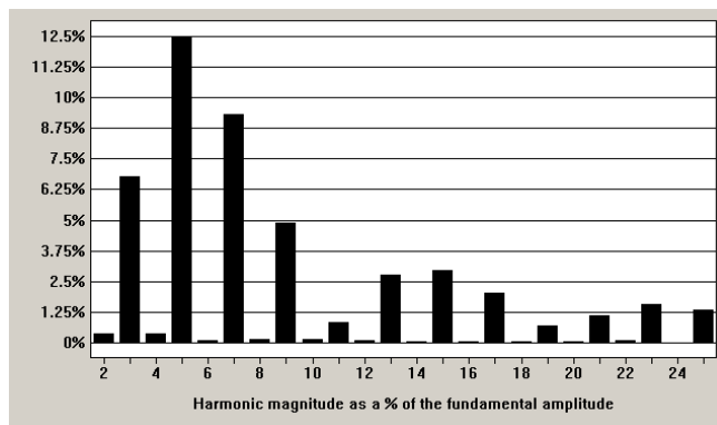
Figura 8. Tablas de análisis espectral y gráficos obtenidos del software WaveStar. Balasto electromagnético. Fuente: elaboración propia.
