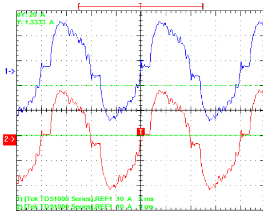
Figura 4. Formas de onda de corriente tomadas sobre dos fases diferentes del tablero de distribución. Fuente: elaboración propia.
