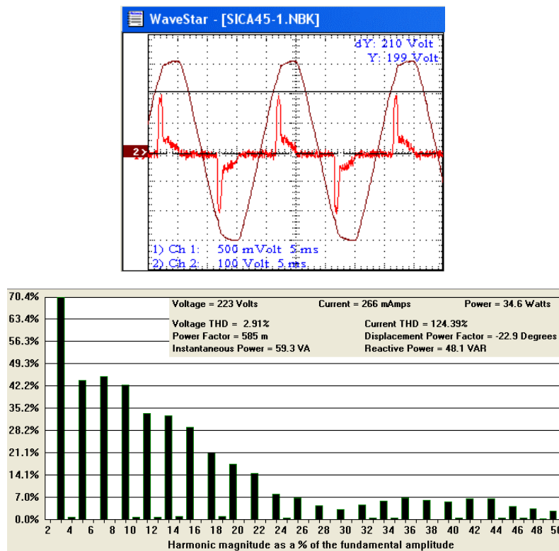
Figura 2. Formas de onda de tensión y corriente correspondiente a una lámpara de bajo consumo. Diagrama de contenido armónico para un THD de 124 % con un coseno phi de -0,92 y un FP = 0,589. Fuente: elaboración propia.
