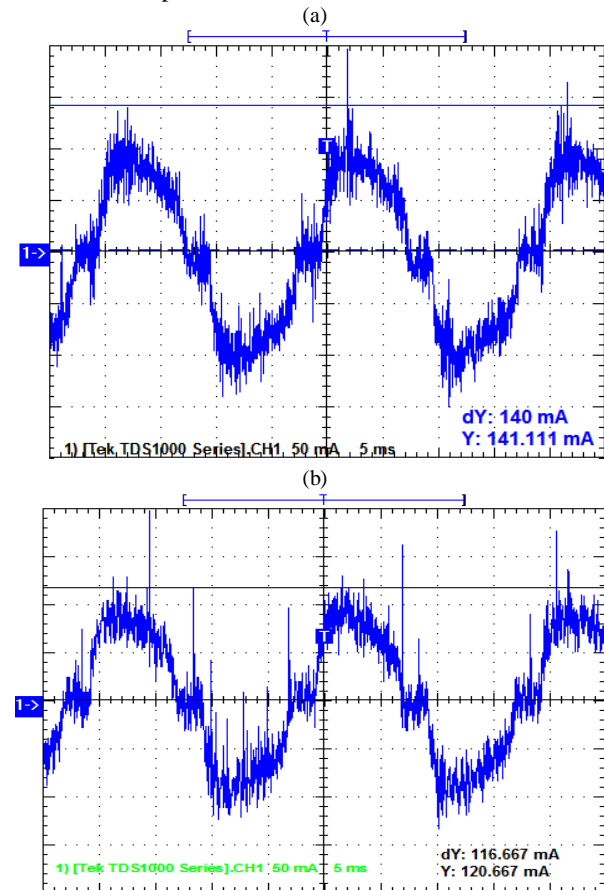
Figura 5. Formas de onda de corriente tomadas en bornes del tubo LED. (a) A los 3 meses de funcionamiento. (b) A los 9 meses. Fuente: elaboración propia.
