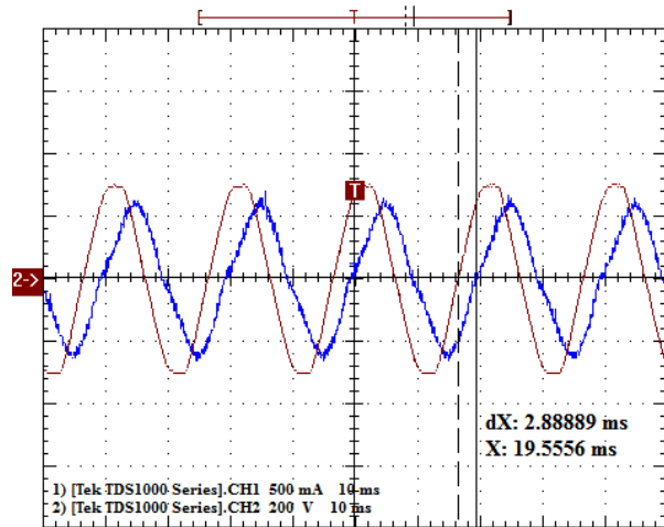
Figura 7. Formas de onda de tensión y corriente para un balasto electromagnético obtenido de la instalación original (año 1968).
