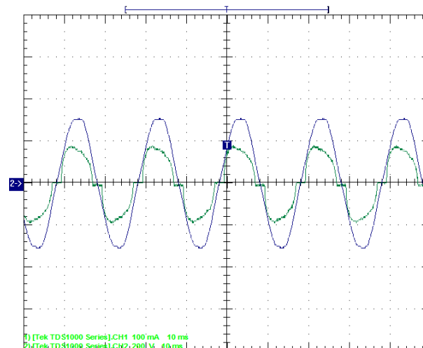
Figura 6. Formas de onda de corriente y tensión tomada en bornes del tubo LED en el laboratorio, en modo de captura promedio del osciloscopio Tektronix 1002B. Fuente: elaboración propia.
