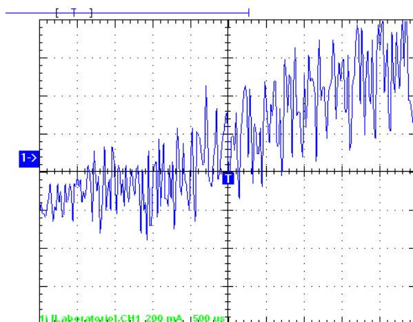
Figura 3. Oscilogramas que muestran la presencia de modulación de HF en corriente de línea de 50 Hz, obtenida con un osciloscopio Tektronix TDS 1002B. Fuente: elaboración propia.
