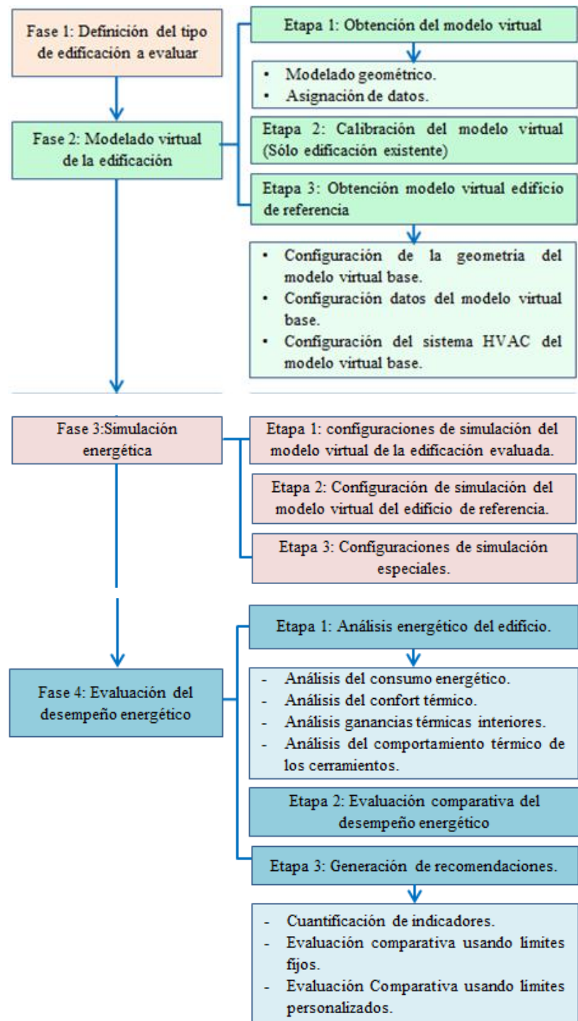
Figura 4. Esquema general de la herramienta metodológica para la evaluación del desempeño energético de edificaciones en el trópico.
