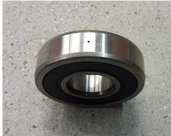
Figura 2. Perforaciones generadas en los rodamientos en la pista exterior. Fuente: elaboración propia.
